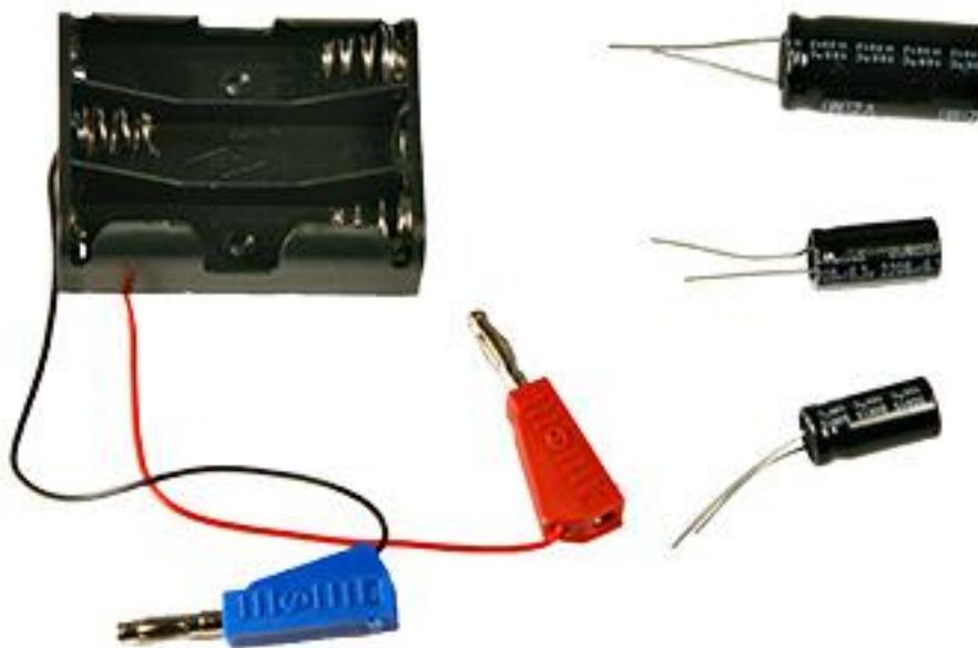
Батарейный блок, электролитические конденсаторы разной емкости.
